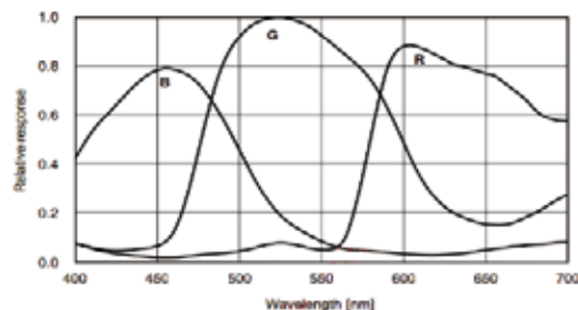
CK-U1200CI-10RS 响应曲线
