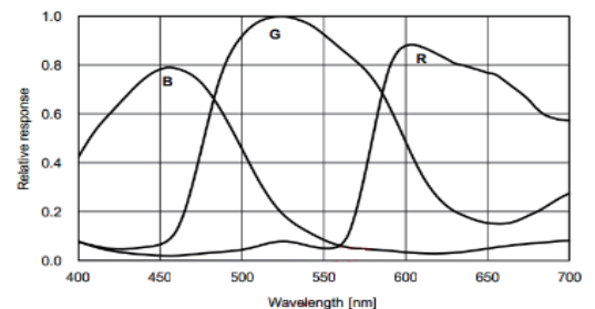
CK-U1200CI-10RS 响应曲线
