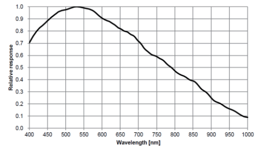
CK-U600MI-19RS 响应曲线
