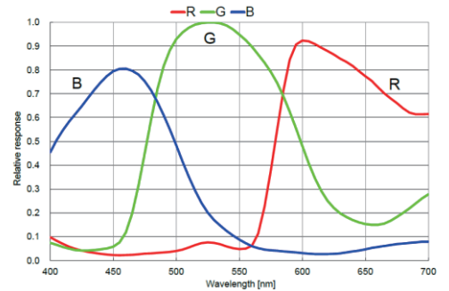
CK-U600CI-19RS 响应曲线
