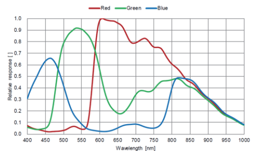
CK-U160CI-66GS 响应曲线
