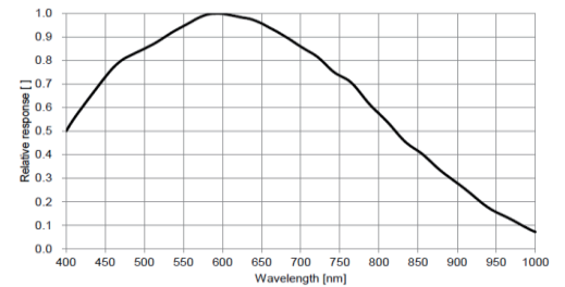
CK-U160MI-66GS 响应曲线
