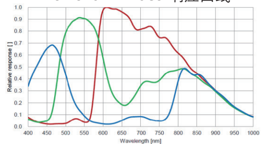
CK-U40CI-126GS 响应曲线
