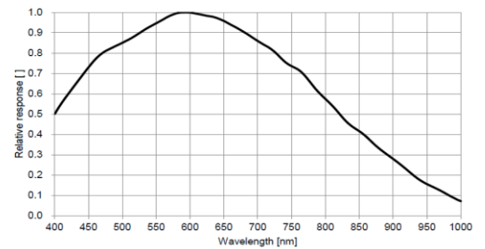
CK-U40MI-126GS 响应曲线
