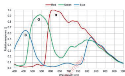
CK-H1200CU-23GS 量子效率
